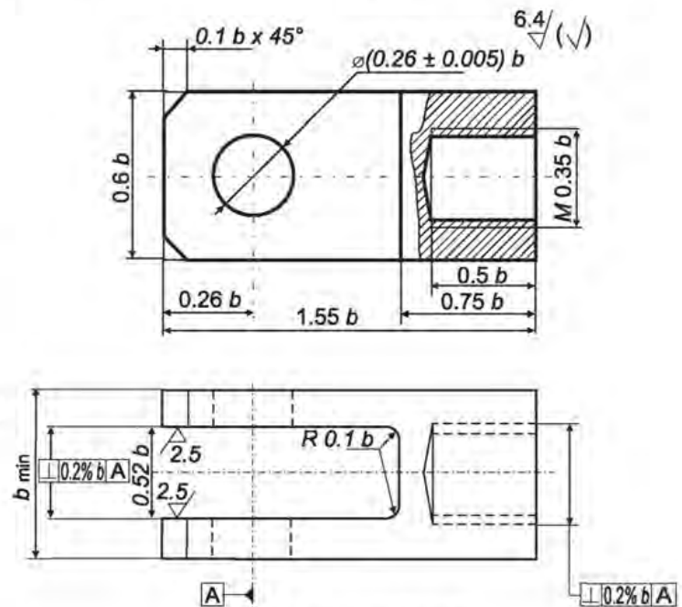
Диаметр пальца 0,25b_{-0,015b}^{-0,005b} Рисунок В.3 — Рекомендуемая конструкция серьги для испытания образцов на внецентренное растяжение.
